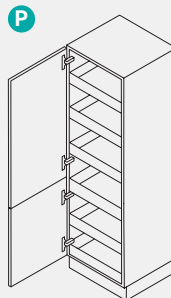
Armoire à provisions d'appoint Hauteur = 1587, 1907, 2051, 2195 mm Largeur = 600 mm 1 porte battante 6 tiroirs à l'anglaise Boční skříň na košťata Výška = 1587, 1907, 2051, 2195 mm Šířka = 600 mm 1 otočné dveře 6 Vnitřní zásuvky
