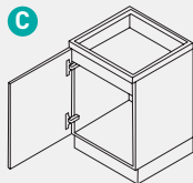
Meuble sous évier Hauteur = 723 mm Largeur = 400, 450, 500, 600 mm 1 porte battante Skříňka pod dřez Výška = 723 mm Šířka = 400, 450, 500, 600 mm 1 otočné dveře
