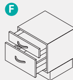
Meuble bas pour machine à laver ou sèche-linge Hauteur = 435 mm Largeur = 600 mm 1 tiroir coulissant 1 tiroir 1 ferrure de sécurité Modul spodní skříňky na pračku nebo sušičku Výška = 435 mm Šířka = 600 mm 1 Výsuvný šuplík 1 Zásuvka 1 Bezpečnostní kování
