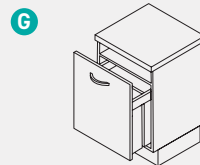
Meuble bas avec système de tri du linge Hauteur = 711 mm Largeur = 600 mm 1 tiroir 2 paniers à linge, 33 litres 1 bac avec couvercle, 20 litres 1 bac, 2,5 litres Spodní skříňka s tříděním prádla Výška = 711 mm Šířka = 600 mm 1 Zásuvka 2 2 koše na prádlo 33 litrů 1 nádoba s víkem, 20 litrů 1 nádoba, 2,5 litrů
