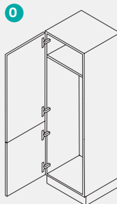
Armoire à balais d'appoint Hauteur = 1587, 1907, 2051, 2195 mm Largeur = 600 mm 1 porte battante 1 tablette fixe Boční skříň na košťata Výška = 1587, 1907, 2051, 2195 mm Šířka = 600 mm 1 otočné dveře 1 pevná police
