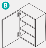
Meuble suspendu Hauteur = 579, 723, 867 mm Largeur = 600 mm 1 porte battante 2 tablettes réglables Závěsná skříňka Výška = 579, 723, 867 mm Šířka = 600 mm 1 otočné dveře Polohovací police
