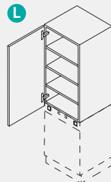
Meuble haut Hauteur = 1181 mm 1 porte battante 3 tablettes réglables Nástavná skříňka Výška = 1181 mm 1 otočné dveře 3 polohovací police
