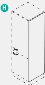
Joues de finition Hauteur = 567, 1097, 2051, 2195 mm Largeur = 585 mm Bočnice Výška = 567, 1097, 2051, 2195 mm Šířka = 585 mm
