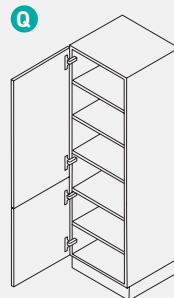
Armoire d'appoint Hauteur = 1907, 2051, 2195 mm Largeur = 600 mm 1 porte battante tablettes réglable 1 tablette fixe Šatní skříň Výška = 1587, 1907, 2051, 2195 mm Šířka = 600 mm 1 otočné dveře polohovací police 1 pevná police
