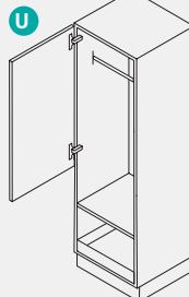
Garde-robe Hauteur = 1907, 2051, 2195 mm Largeur = 600 mm 2 tablettes fixes 1 tringle à vêtements 1 tiroir à l'anglaise Šatní skříň Výška = 1907, 2051, 2195 mm Šířka = 600 mm 2 pevné dno 1 tyč na šaty 1 vnitřní zásuvka
