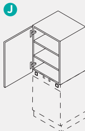
Meuble haut Hauteur = 717 mm 1 porte battante 2 tablettes réglables Nástavná skříňka Výška = 717 mm 1 otočné dveře 2 polohovací police
