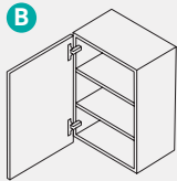
Hängeschränk Höhe = 579, 723, 867 mm Breite = 600 mm 1 Drehtür verstellbarer Fachboden Wall cabinet Height = 579, 723, 867 mm Width = 600 mm 1 swing door Adjustable shelves
