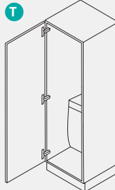
HWR Schrank mit Ordnungssystem Höhe = 1907, 2051, 2195 mm Breite = 600 mm 1 Wertstoffdepot mit Baumwollsaack 1 Ablage mit Kehrlech 2 Bügelbretthalter Utility room cupboard with in-built organiser Height = 1907, 2051, 2195 mm Width = 600 mm 1 recycling bin with cotton bag 1 shelf with dustpan 2 ironing board holders
