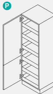
Seitenschrank für Vorräte Höhe = 1587, 1907, 2051, 2195 mm Breite = 600 mm 1 Drehtür 6 Innenschubkästen Side pantry cabinet Height = 1587, 1907, 2051, 2195 mm Width = 600 mm 1 swing door 6 internal drawers
