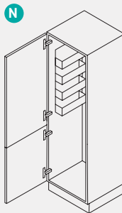
Seitenschrank für Besen Höhe = 1587, 1907, 2051, 2195 mm Breite = 600 mm 1 Drehtür 1 Drahtregal 3 Haken für Besen 1 Universalhalter Tall cabinet for brooms Height = 1587, 1907, 2051, 2195 mm Width = 600 mm 1 swing door 1 metal storage rack 3 broom hooks 1 universal holder
