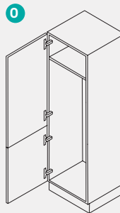
Seitenschrank für Besen Höhe = 1587, 1907, 2051, 2195 mm Breite = 600 mm 1 Drehtür 1 fester Fachboden Side cabinet for brooms Height = 1587, 1907, 2051, 2195 mm Width = 600 mm 1 swing door 1 fixed shelf
