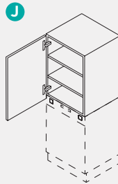
Aufsatzschrank Höhe = 717 mm 1 Drehtür 2 verstellbare Fachböden Top-mounted cabinet Height = 717 mm 1 swing door 2 adjustable shelves
