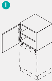
Aufsatzschrank Höhe = 573 mm 1 Drehtür 1 verstellbarer Fachboden Top-mounted cabinet Height = 573 mm 1 swing door 1 adjustable shelf
