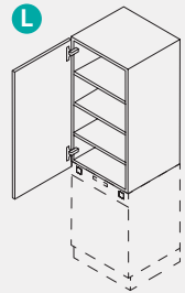
Aufsatzschrank Höhe = 1181 mm 1 Drehtür 3 verstellbare Fachböden Top-mounted cabinet Height = 1181 mm 1 Swing door 3 adjustable shelves
