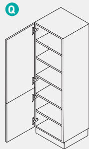
Seitenschrank Höhe = 1587, 1907, 2051, 2195 mm Breite = 600 mm 1 Drehtür verstellbare Fachböden 1 fester Fachboden Side cabinet Height = 1587, 1907, 2051, 2195 mm Width = 600 mm 1 swing door adjustable shelves 1 fixed shelf
