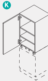
Aufsatzschrank Höhe = 861 mm 1 Drehtür 2 verstellbare Fachböden Top-mounted cabinet Height = 861 mm 1 Swing door 2 adjustable shelves
