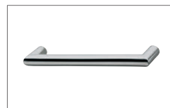
N° 852 Poignée arc métallique aspect inox Profondeur 40 mm Entraxe perforations : 160 mm
