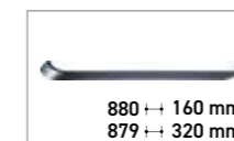
880*/879*** Poignée arc métallique graphite 880*/879*** Metalen beugelgreep grafiet
